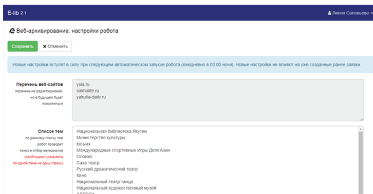
Рис. 2. Веб-интерфейс «Веб-архивирование: настройки работы»
